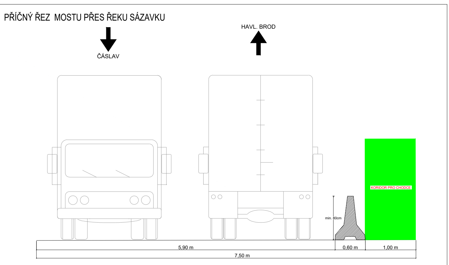
DETAIL HABRY - MOST PŘES ŘEKU SÁZAVKU
